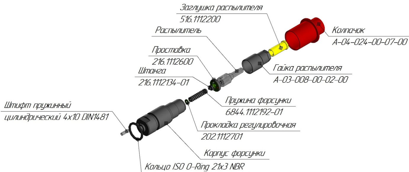
Рисунок 1 – Комплектующие форсунок А-03-008-00-00-00...08
