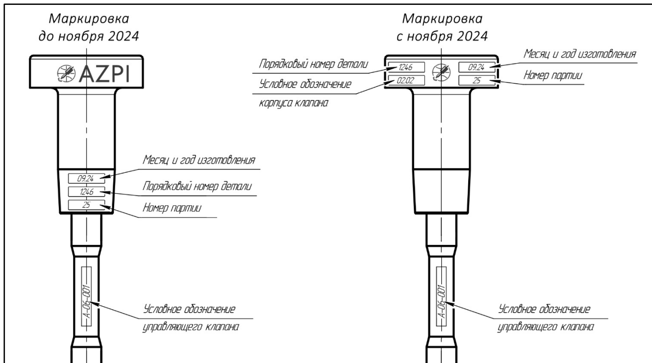
Рисунок 2 – Управляющие клапаны поставляемые на вторичный рынок запасных частей.
