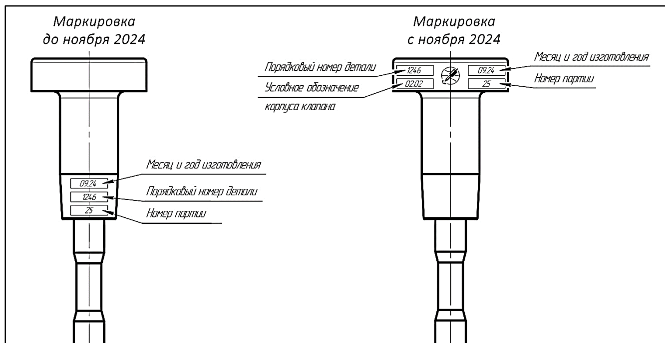
Рисунок 1 – Управляющие клапаны поставляемые на конвейеры в составе инжекторов CR.
