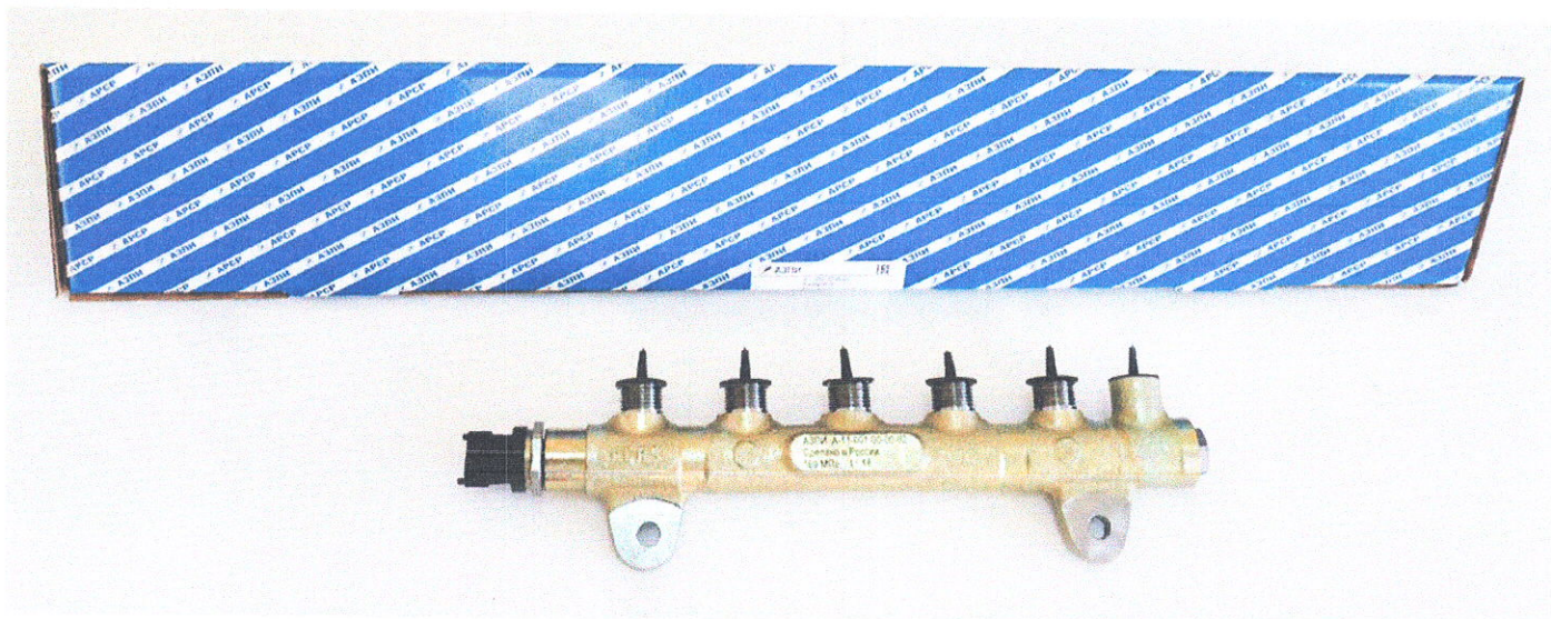
Рисунок 1 - Топливный аккумулятор A-11-001-00-00-02 (аналог 0445224047)
